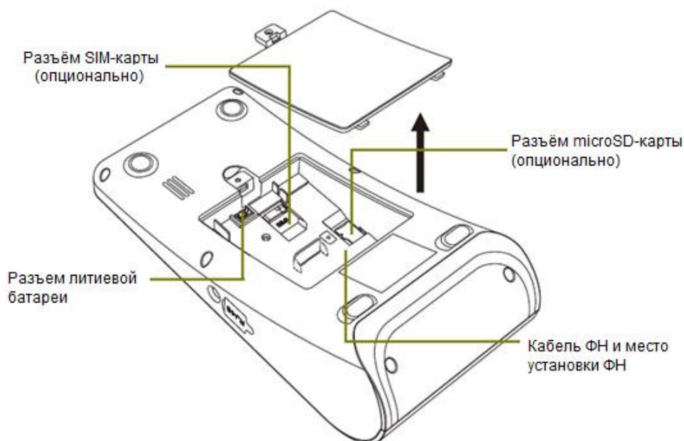
Рис. 2 Отсек литиевой батареи и ФН
