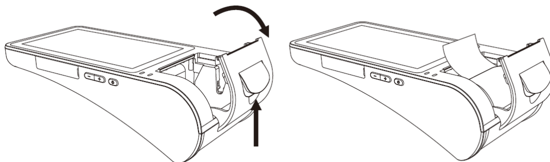
Рис. 4 Заправка бумаги
